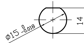
C 矢視図
