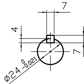
C 矢視図
