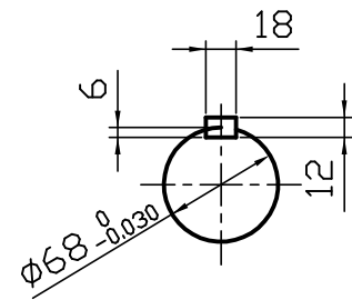
C 矢視図
