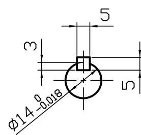
A 矢視図
