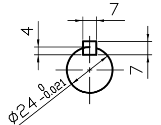
C 矢視図 D 矢視図
