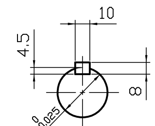
C 矢視図 D 矢視図
