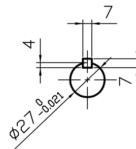
A 矢視図
