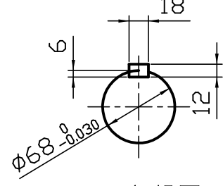
C 矢視図
