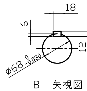
C 矢視図
