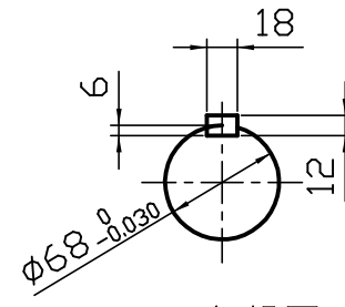
C 矢視図
