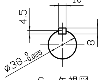
C 矢視図
