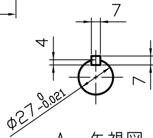
A 矢視図
