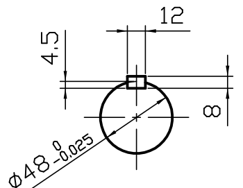
B 矢視図
