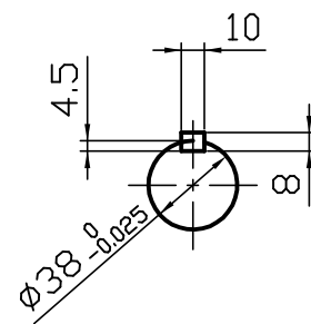
C 矢視図
