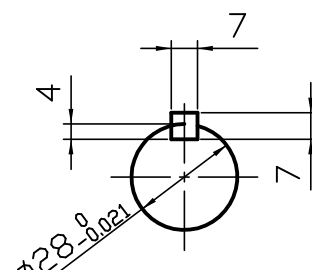
B 矢視図
