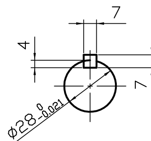
C 矢視図
