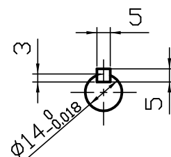
A 矢視図
