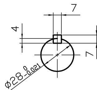
C 矢視図
