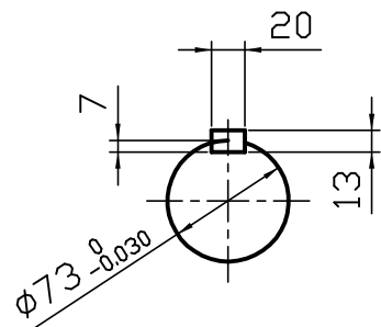
C 矢視図
