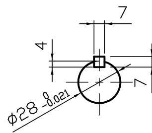
B 矢視図
