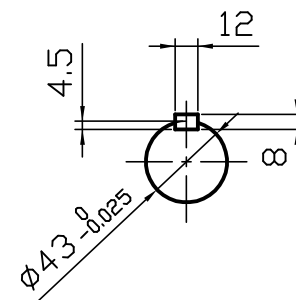
C 矢視図 D 矢視図
