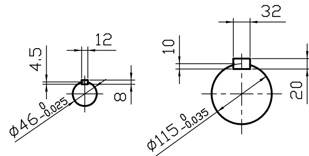
A 矢視図 B 矢視図 C 矢視図
